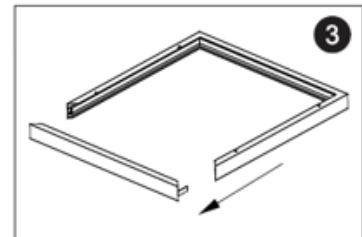
3. Afmonter nu den side af rammen, der ikke har montagehuller - som vist herover
