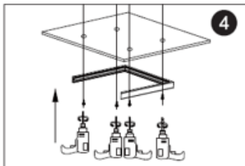
4. Monter rammens 3 sider på loftet med skruer
