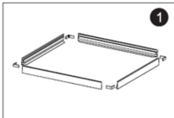
1. Monter de 4 samlebeslag i rammen
