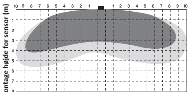
Detektionsmønster ved loftmontage (m)
